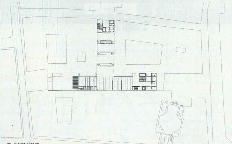
39 · PLANTA SÓTANO
